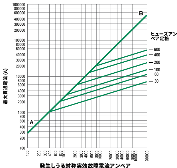
図7 - 最大貫通電流チャート
