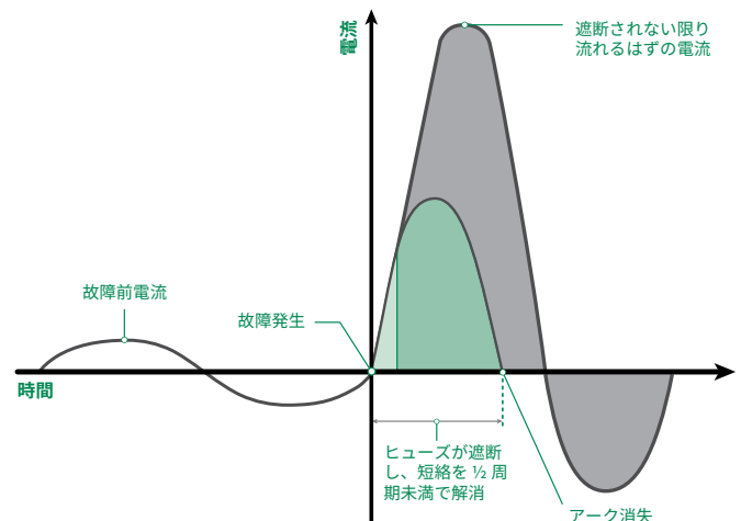
図 13 - 電流制限ヒューズ
