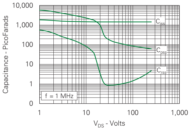
Fig. 11. Capacitance
