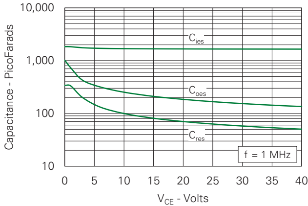
Fig. 9. Capacitance
