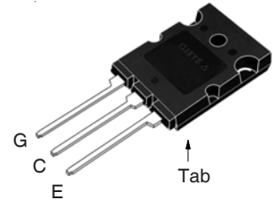
PLUS247 (IXYX)
