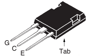
PLUS247 (IXYX)
