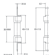
ZXPY Blade
